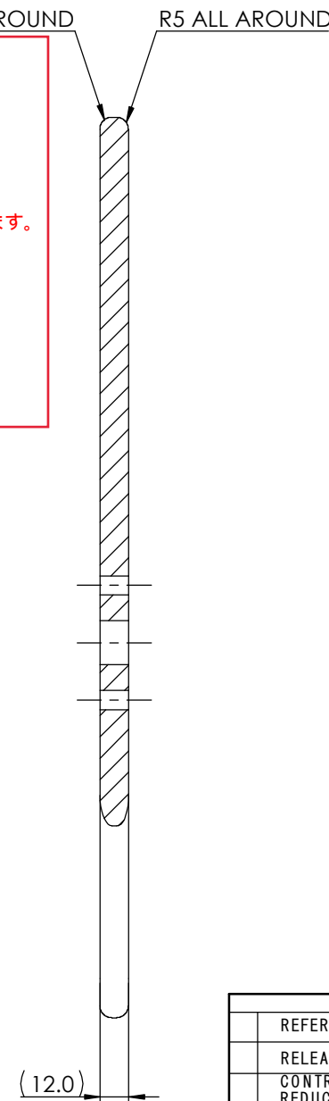
断面図 A-A
