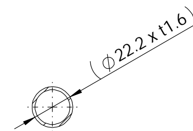
断面図 A-A
