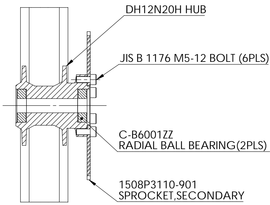
断面図 A-A スケール 1 : 2
