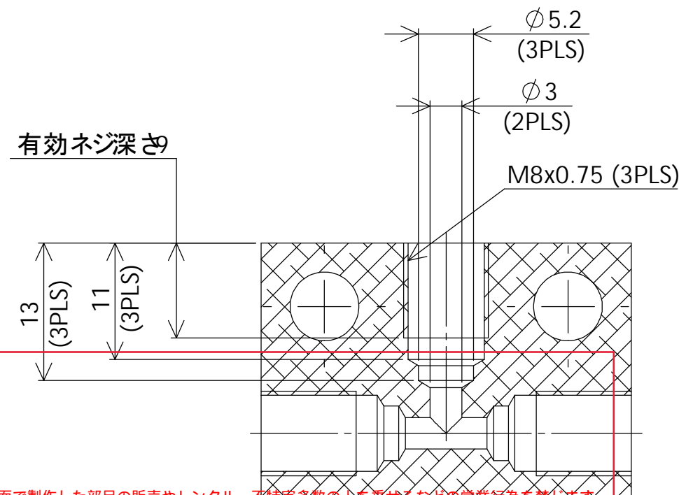
断面図 A-A
